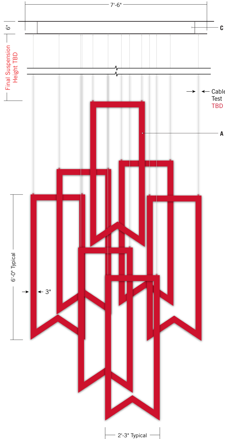
FRONT VIEW Scale: 1/2" = 1'- 0" QTY: 7
